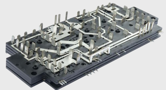
Stanzgitter
